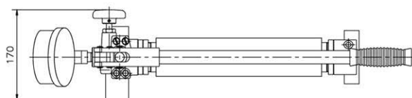
HML-1700N/2000N 寸法図
